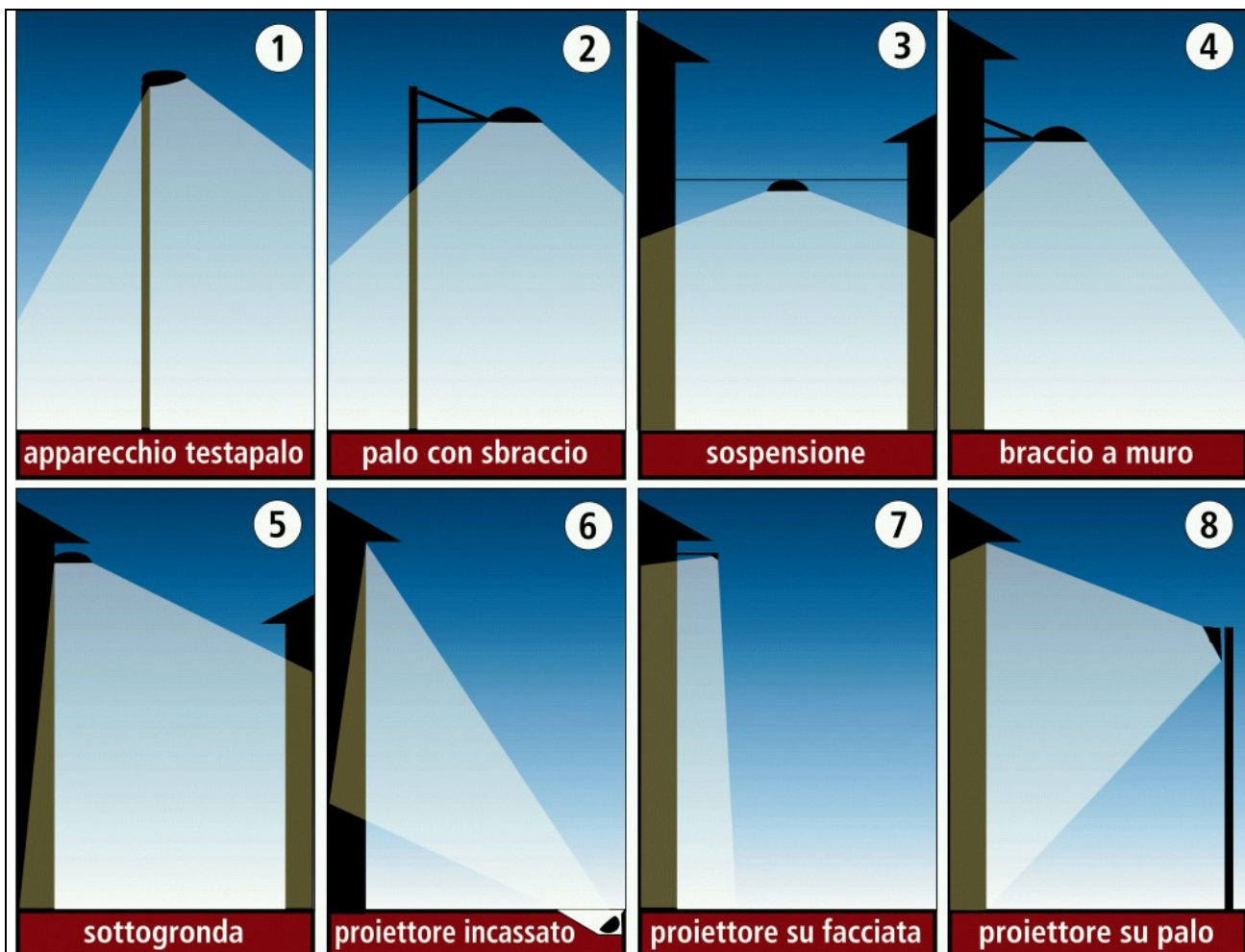
Figura 2.6 – Apparecchi conformi alla L.r. 17/00 e s.m.i.. Le tipologie 6 e 8 sono ammesse esclusivamente per l’illuminazione di edifici storici a di alto valore architettonico ove non possa essere fatto altrimenti. (Cortesia: CieloBuio)
