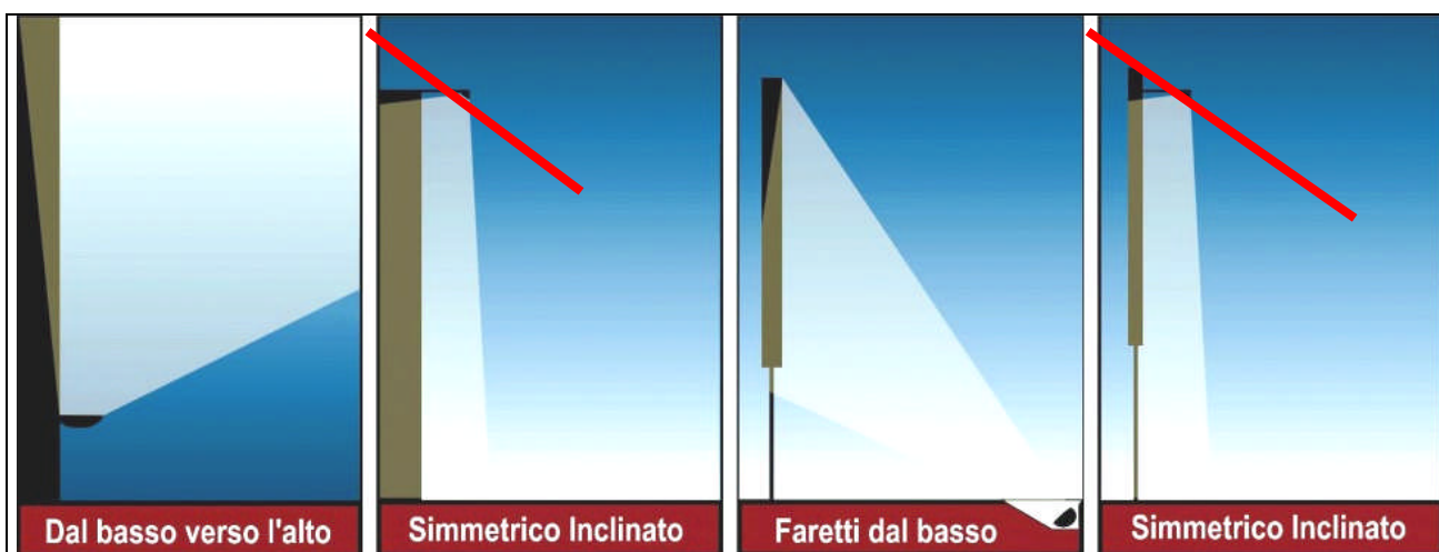
Figura 2.16 – Installazioni non conformi alla L.r. 17/00 e s.m.i.. Partendo da sinistra l'illuminazione dal basso non è consentita se non per illuminazione di manufatti storici ed artistici ma mantenendo il fascio all'interno della sagoma dello stesso, nella seconda l'illuminazione dell'apparecchio inclinato va oltre l'edificio in quanto il piano passante per il vetro del proiettore inclinato non viene intercettato dalla parete. Nella terza e quarta immagine l'illuminazione del cartellone non è corretta in quanto l'unica illuminazione corretta sarebbe con proiettore orizzontale dall'alto verso il basso. (Cortesia CieloBuio)
